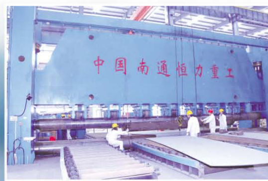
■ 1200t 船用卷板机 1200t roll plate bending machine
